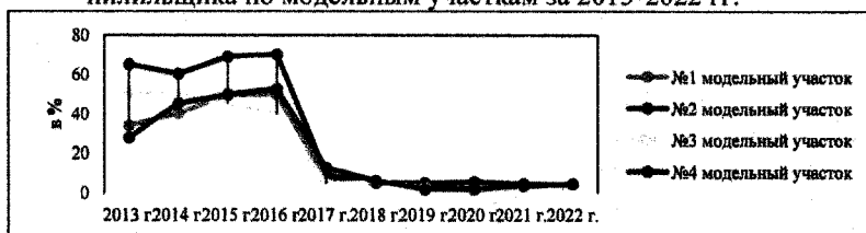
Диаграмма 3.3.1.2- Динамика численности вязового минирующего пилильщика по модельным участкам за 2013-2022 гг.
