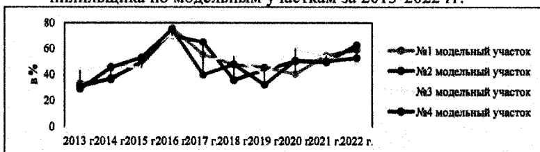
Диаграмма 3.3.1.3- Динамика численности каштановой минирующей моли по модельным участкам за 2013-2022 гг.
