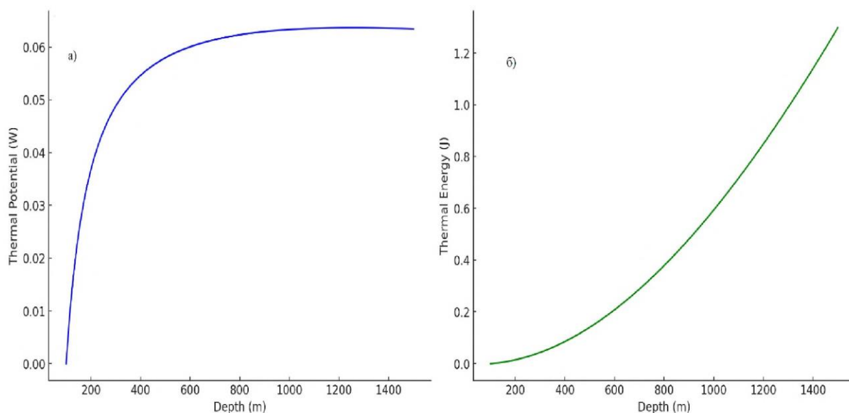
Рис. 1. Зависимость теплового потенциала ( P(h) ) и накопленной тепловой энергии ( E(h) ) от глубины скважины для геотермальных источников города Джалал-Абад, Кыргызская Республика.
