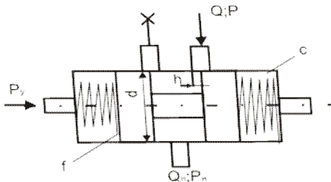
Рис.5 Расчетная схема
