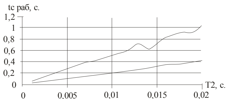
Рис. 9 График зависимости времени переходного процесса от T_2 при различных \xi_2
