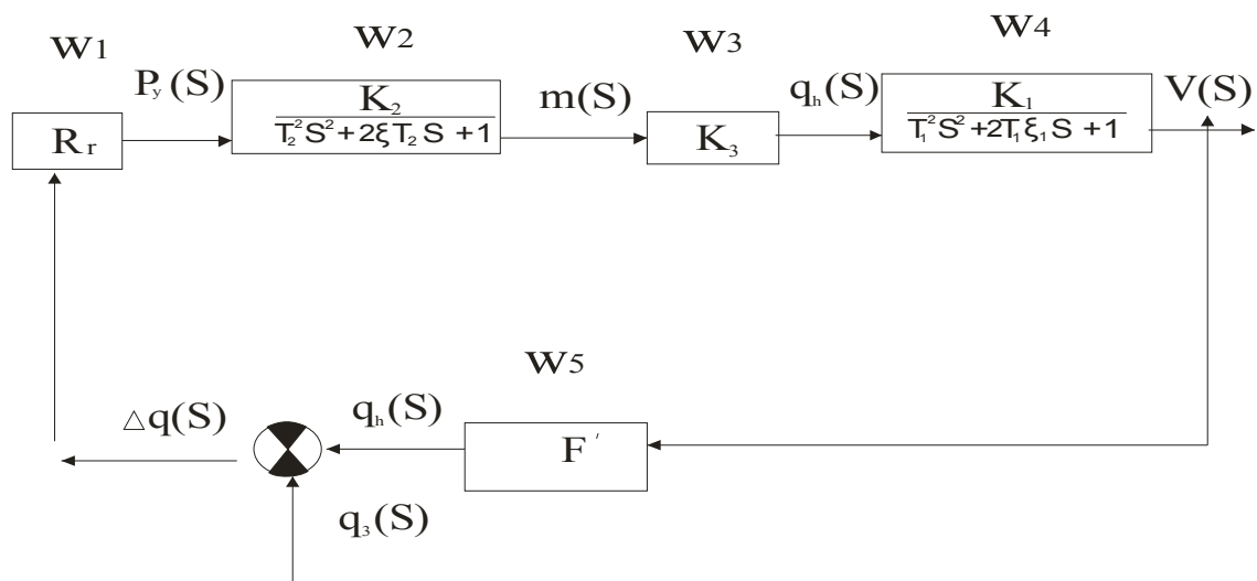
Рис. 7 Структурная схема гидропривода с обратной гидравлической связью
