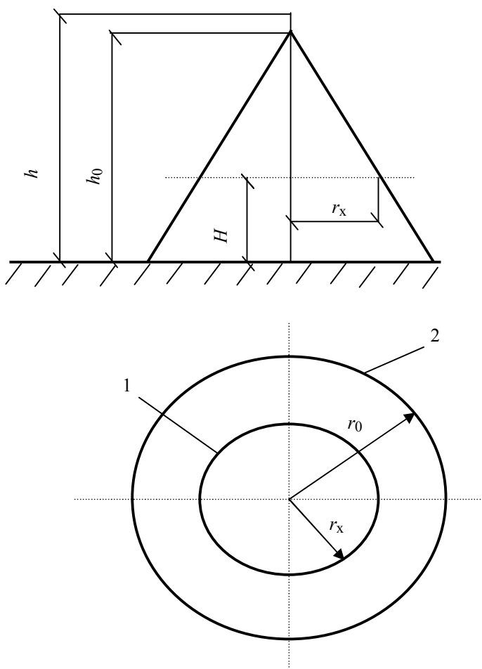
Рис. 14.1. Зона защиты одиночного стержневого молниеотвода: 1 – граница зоны защиты на уровне высоты объекта; 2 – то же, на уровне земли; h – высота молниеотвода; h_0 – высота конуса защиты; H – высота защищаемого объекта; r_x – радиус зоны защиты на уровне высоты объекта; r_0 – радиус зоны защиты объекта на уровне земли.
