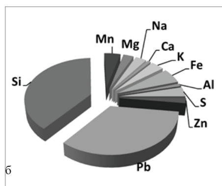
Рисунок 7 – Поэлементный состав полученных образцов дистиллятов (а) и остатков (б), полученных при T\ 1100\ ^\circ\text{C} в инертно-восстановительной атмосфере
