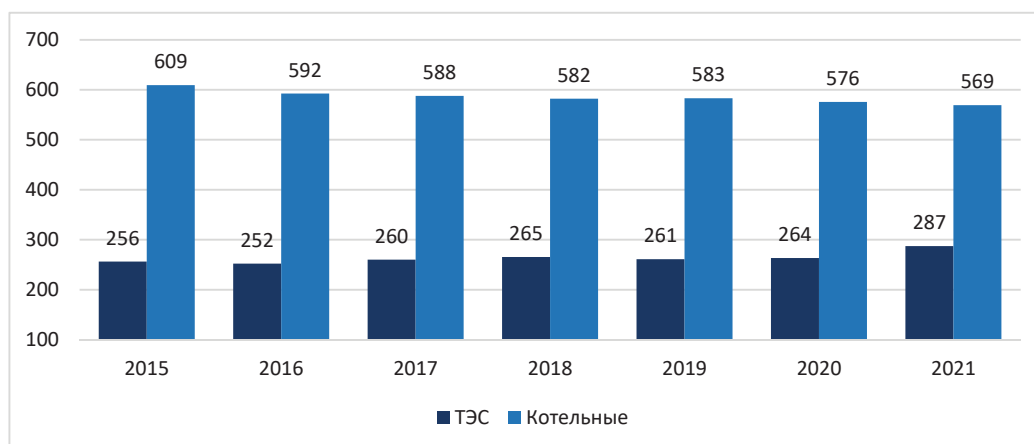
Рисунок 2 – Суммарная мощность по видам источников теплоснабжения в 2015–2021 гг., тыс. Гкал/час
