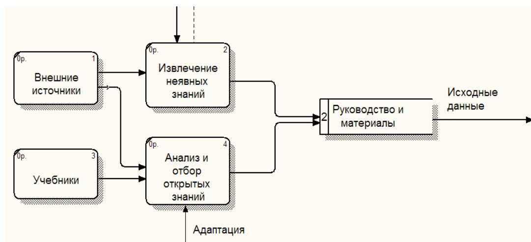
Рисунок 2 – Детализация блока “Добывание знаний”
