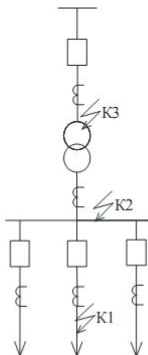
Рис.1. Схема подстанции
