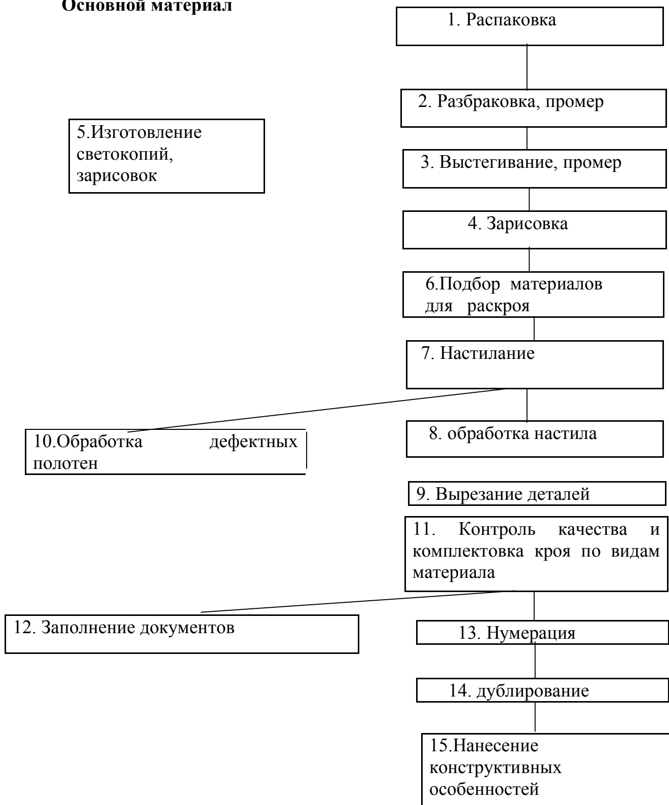
Рис.1 Укрупненный граф ТП подготовительно-раскройного производства.
