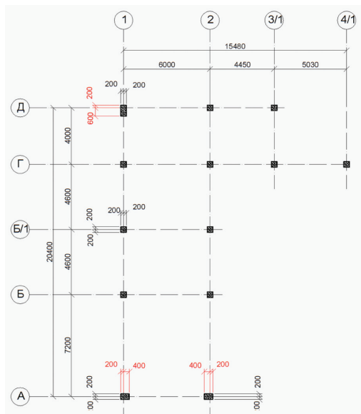
Рис. 4. Схема колонн для схемы 4
