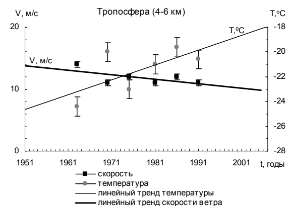
Рис. 2. Временные вариации температуры воздуха T(t) и зональной компоненты скорости ветра V(t) .
