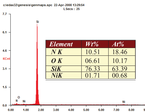
Рис. 2. Результаты локального микрорентгеноспектрального анализа включений, имеющих в структуре реакционно-спечённого НККМ: а – поверхность излома спечённого образца при T=1320^{\circ}\text{C} . Локально отснят спектр с криволинейного нитевидного кристалла (верхняя левая угловая точка Spectrum 6). Спектр и содержание элементов в данной точке представлены в виде таблицы; б – поверхность шлифа (крестиком отмечена частица, с которого произведен анализ).
