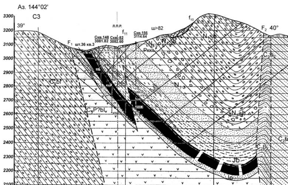
Рис. 3. Геологический разрез месторождения Кара-Кече по профилейной линии 11.
