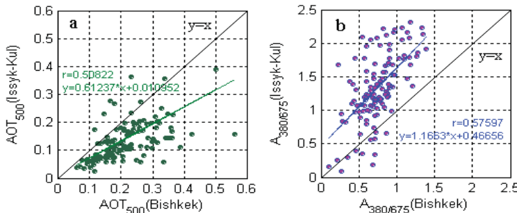
Рис. 6. Сопоставление результатов измерения AOT 500 (а) и расчета параметра A_{380/675} (б) для Issyk-Kul и Bishkek_Site. Май-сентябрь 2008 г.
