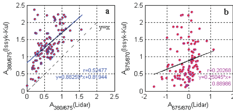
Рис. 5. Сопоставление результатов вычисления параметров A_{380/675} и A_{675/870} для данных Issyk-Kul и LidarSite. Май-сентябрь 2008 г.
