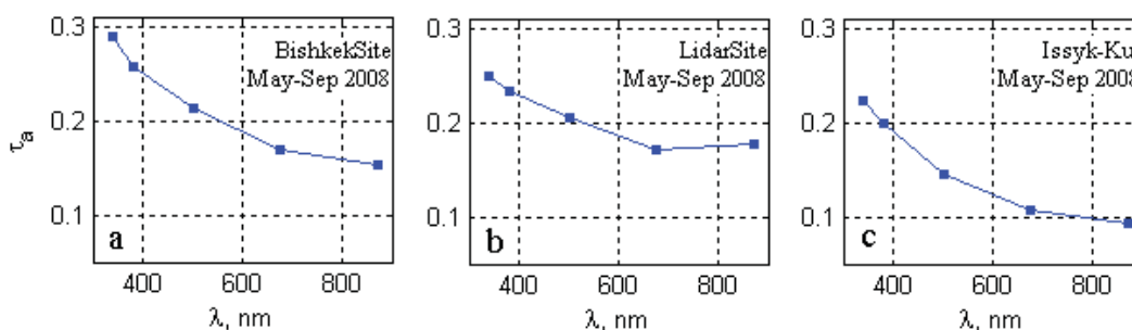
Рис. 7. Средние спектральные зависимости АОТ на трех пунктах контроля. Май-сентябрь 2008 г.
