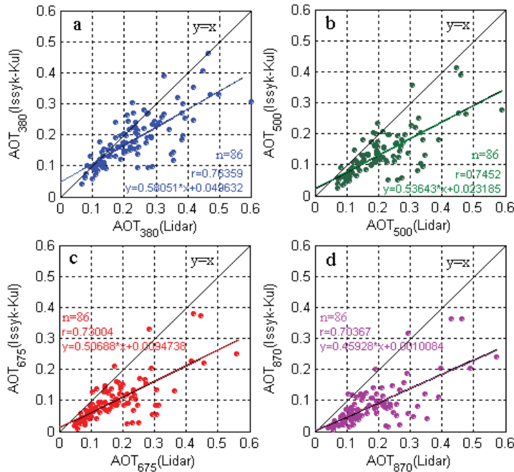
Рис. 4. Сопоставление результатов измерения AOT на длинах волн 380, 500, 675 и 870 нм на Issyk-Kul и LidarSite. Май-сентябрь 2008 г.
