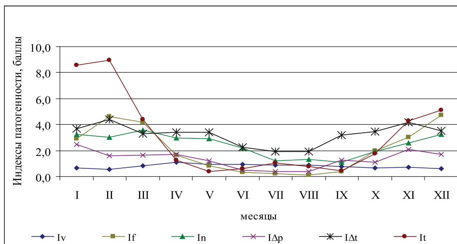
Рис. 2. Годовой ход частных индексов I_x по станции Бишкек.
