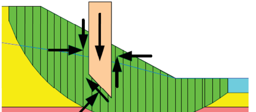
Рис. 1. Силы, действующие на блок.
