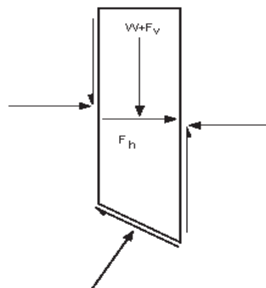
Рис. 2. Псевдосейсмические силы, действующие на блок.
