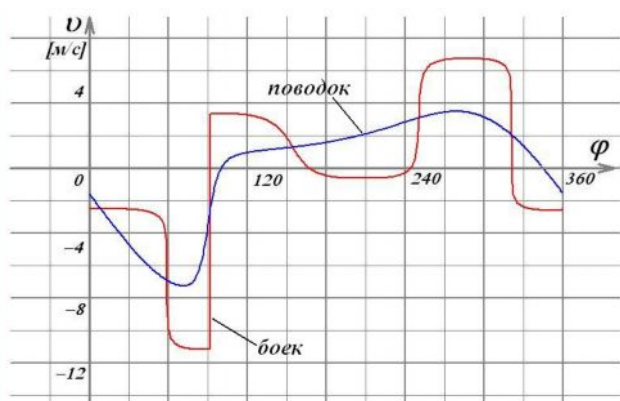
Рис. 5. Графики скорости бойка на оборотах с 11 по 20 при k_{отс}=0,3 .
