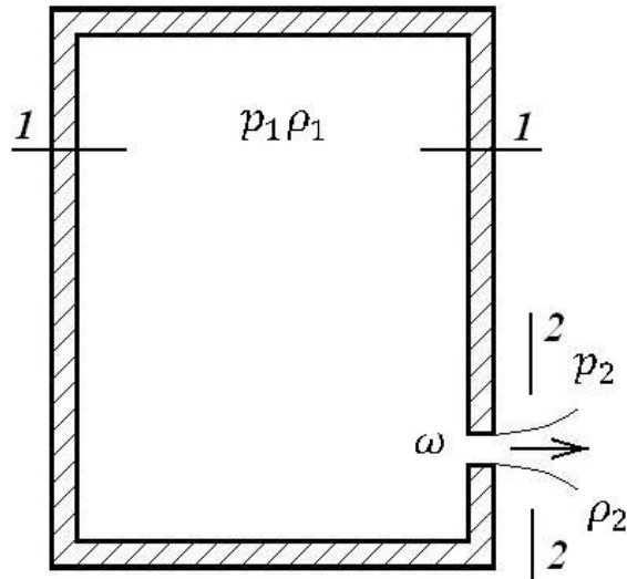
Рис. 2. Истечение газа из отверстия в тонкой стенке
