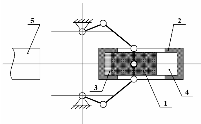
Рис.1. Схема возникновения воздушной подушки при рабочем ходе:
