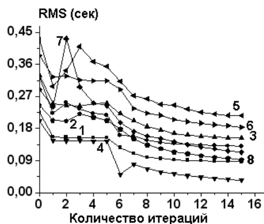
Рис. 3. Изменения RMS как функции итерационного процесса для восьми наибольших кластеров.
