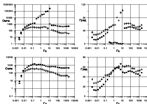
Рис. 5. Кривые кажущегося сопротивления и фазы импеданса для пункта Чон-Курчак (вверху – стандартная обработка, внизу – углубленная).
