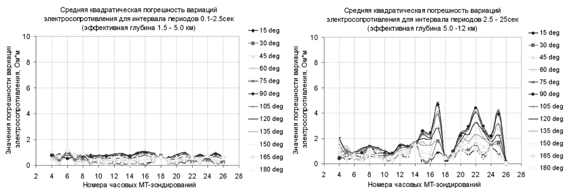
Рис.7. Распределение среднеквадратического отклонения от среднего для ориентированных кривых вариаций электропроводности между двумя станциями Phoenix MTU-5D №1571 и №1918.
