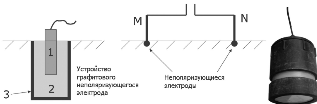
Рис. 2. Измерение горизонтальных компонент электрического поля.
