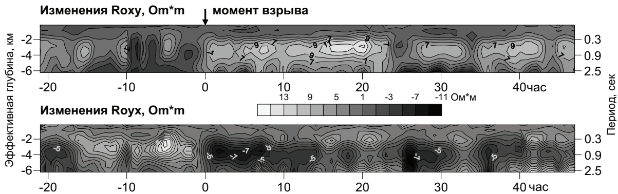
Рис. 10. Временные ряды вариаций компонент тензора импеданса по Камбаратинскому эксперименту, представленные в виде псевдоразрезов кажущегося сопротивления по направлениям ху и ух, (т.е. азимуты 0 и 90°).
