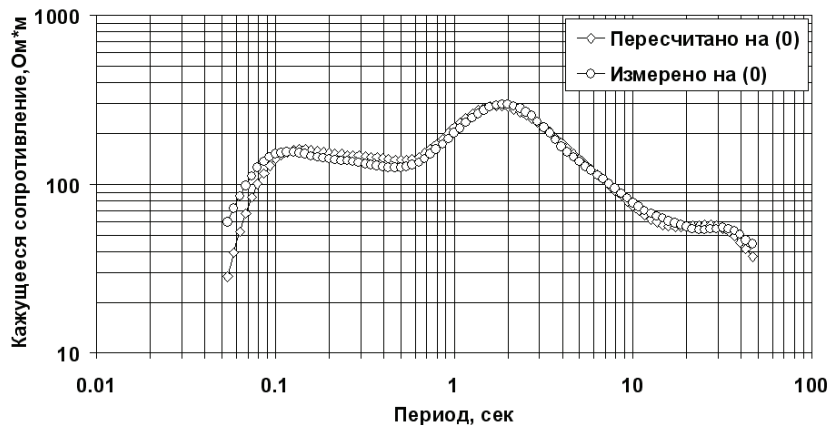
Рис. 13. Сопоставление кривых кажущегося сопротивления, измеренных по азимуту 0^\circ с кривыми, измеренными на азимуте -45^\circ и пересчитанными на азимут 0^\circ .
