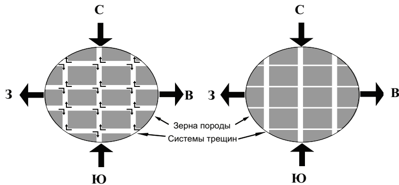
Рис. 12. Феноменологическая модель перераспределения флюида между системами трещин при изменении напряженно-деформационного состояния среды. Толстыми стрелками показаны направления действия силы сжатия и растяжения.
