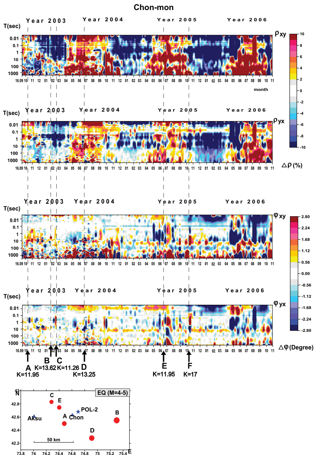
Рис. 9. Пункт мониторинга Чон-Курчак. Отклонения среднесуточных оценок обеих мод амплитуд и фаз кажущегося сопротивления от средних кривых. Отклонения нормированы на средние оценки за весь период анализа и выражены в процентах.
