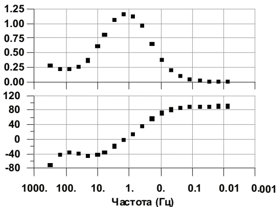
Рис. 4. Амплитудно-фазовая частотная характеристика магнитного канала MTU-5D с индукционным датчиком МТС-50 (вверху – амплитуда в усл. ед., внизу – фаза в град.)
