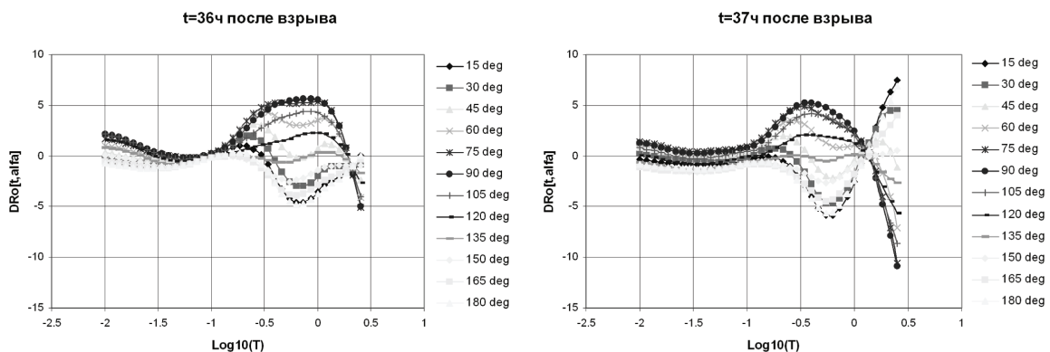
Рис. 11. Пример семейств ориентированных кривых кажущегося сопротивления DRo_{[t,\alpha]} во время Камбаратинского эксперимента для 36 и 37-го часа после взрыва: t=36 , t=37 , \alpha от 15 до 180°; Т – период МТ-зондирования.
