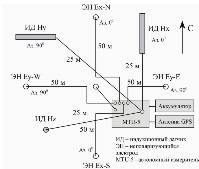
Рис. 3. Измерительная установка пяти компонент МТ поля с использованием станции Phoenix MTU-5D.
