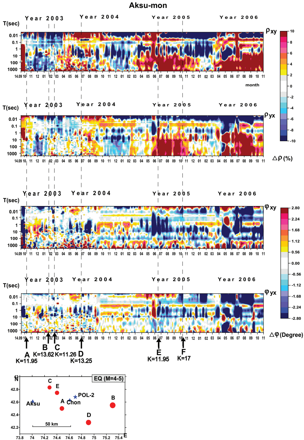
Рис. 8. Пункт мониторинга Аксу. Отклонения среднесуточных оценок обеих мод амплитуд и фаз кажущегося сопротивления от средних кривых. Отклонения нормированы на средние оценки за весь период анализа и выражены в процентах.
