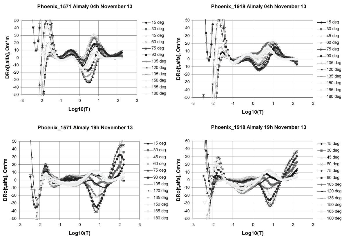
Рис. 6. Результаты контрольных измерений для определения точности оценки азимутальных характеристик вариаций электропроводности на пункте Алмалы (для 4-й и 19-й часовых реализаций).
