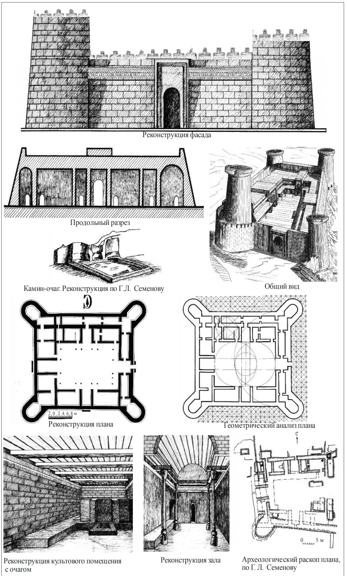
Рис. 2. Цитадель-дворец в Суябе. Вариант реконструкции О. Воличенко, Ж. Казиева
