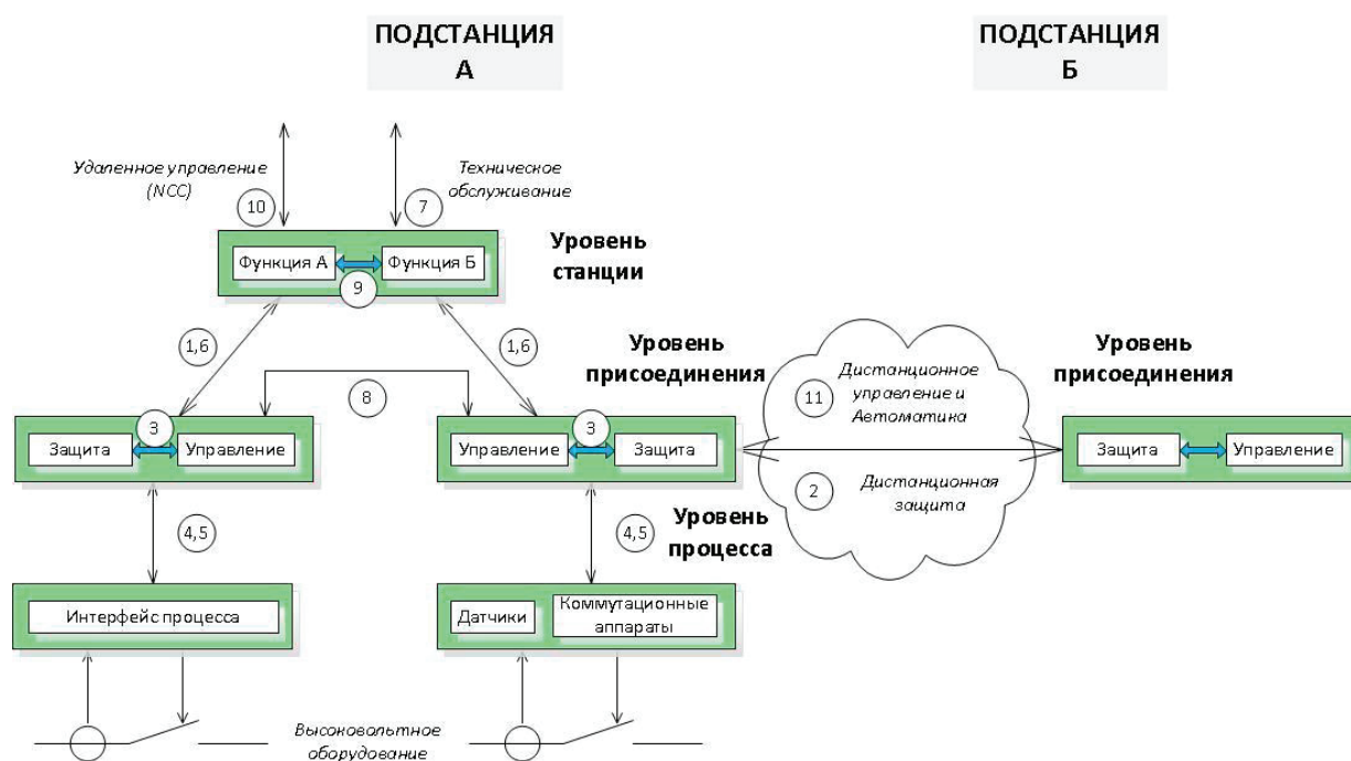
Рисунок 2 – Архитектура системы связи цифровой подстанции [4]
