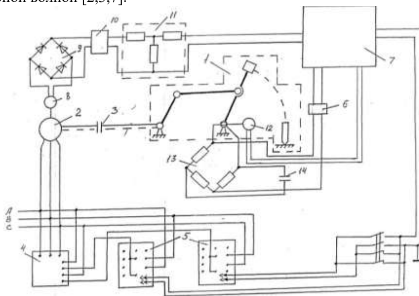
Рис. 1. Экспериментальный стенд
