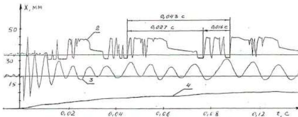
Рис. 3. Диаграммы усилия 2, потребляемой мощности электродвигателя 3, угловой скорости электродвигателя 4
