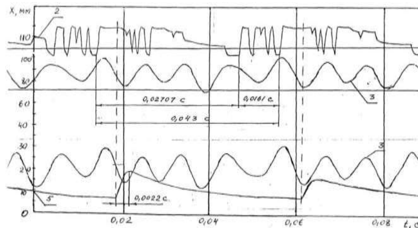
Рис. 4. Диаграммы усилия 2, потребляемой мощности электродвигателя 3 и контактов 5
