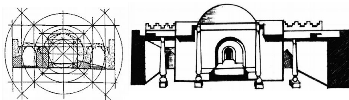
Рис. 2. Разрез первого буддийского храма. Анализ геометрических пропорций, по С. Я. Перегудовой
