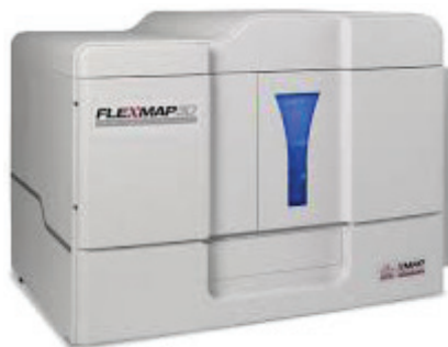
Рисунок 25 – Luminex xMAP
