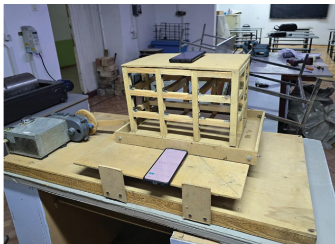
Рисунок 1 – Общий вид стенда в процессе испытаний модели
