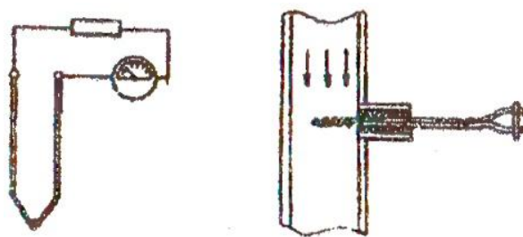
Рис. 12. Схема устройства для определения температуры отработавших газов с использованием термопары
