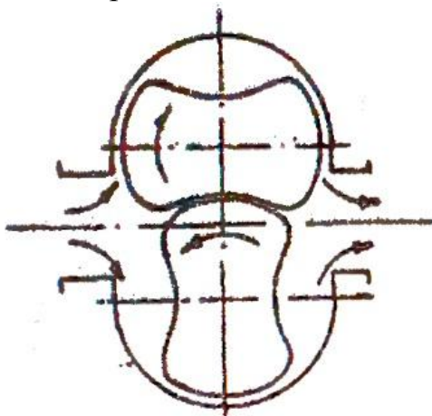
Рис. 9. Схема объемного расходомера воздуха
