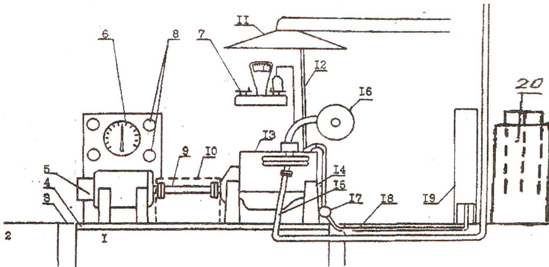
Рис. 6. Испытательный стенд: 1-фундамент стенда; 2-фундамент здания; 3-настил; 4-подмоторная рама; 5-тормоз; 6-весовой механизм; 7-устройство для определения расхода топлива; 8-приборы (тахометр, указатель температуры охлаждающей жидкости, указатель давления масла, указатель температуры масла); 9-соединительный вал; 10-защитный кожух; 11-зонт системы вентиляции; 12-шланг для отвода картерных газов; 13-двигатель; 14-стойка; 15-выхлопная труба; 16-устройство для измерения расхода воздуха; 17-устройство для измерения расхода охлаждающей жидкости; 18-канал со шлангами и выхлопной трубой; 19-смеситель охлаждающей жидкости; 20-жидкостный реостат
