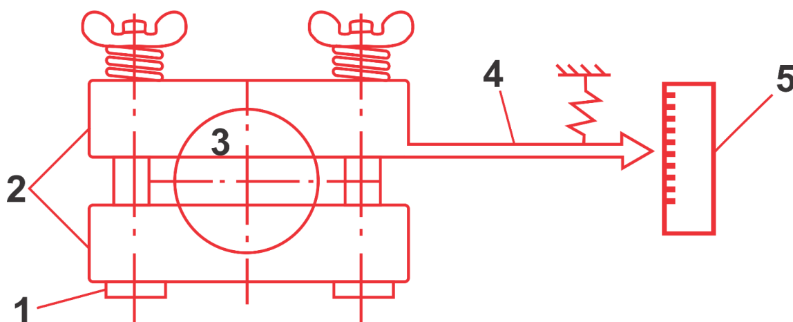
Рис.1. Схема механического тормоза: 1 - стяжные болты; 2 - колодка; 3 - барабан; 4 - весы; 5 - шкала.
