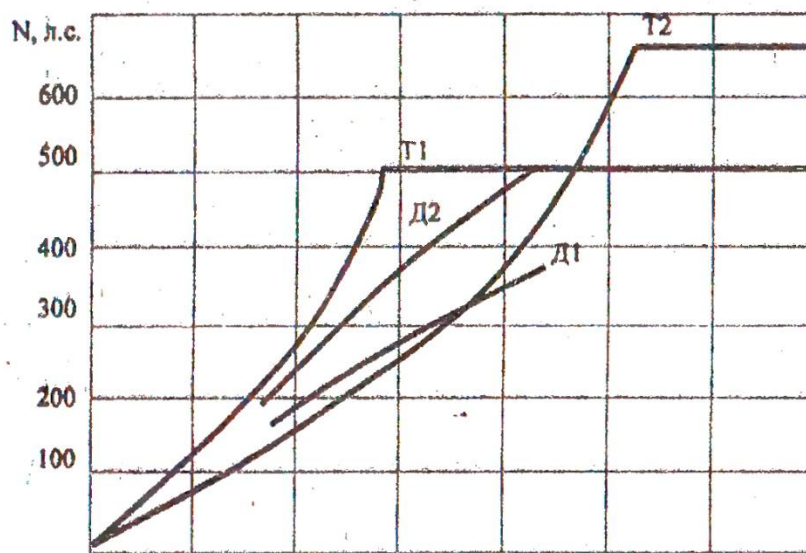
Рис. 5. Сопоставление скоростных характеристик двигателя и тормоза.
