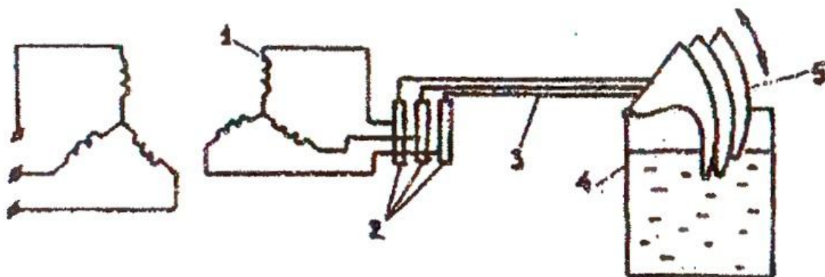
Рис. 2. Схеме системы регулирования электрического тормоза жидкостным реостатом: 1 - обмотка ротора; 2 - контактные кольца; 3 - соединительные провода; 4 - нагрузочный реостат; 5 - пластины реостата.
