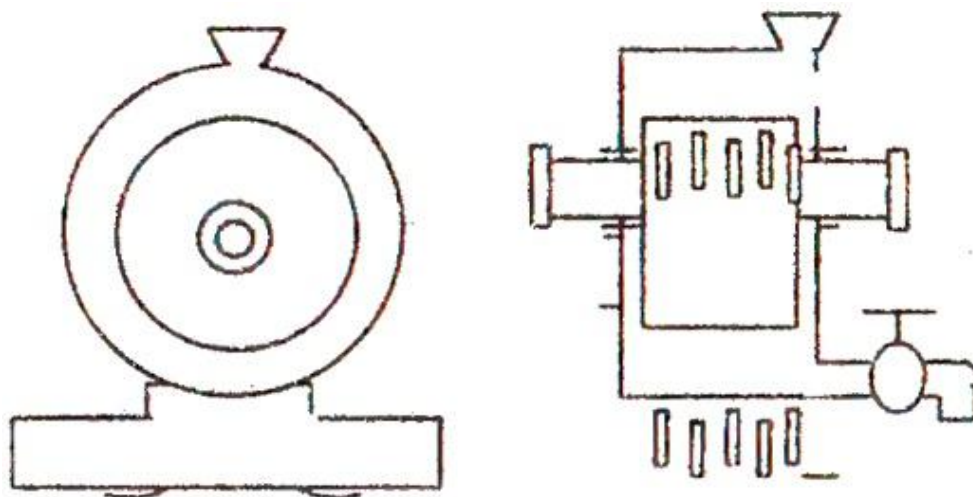
Рис. 3. Схем» гидравлического тормоза штифтового типа.
