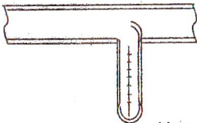
Рис. 10. Изменение расхода воздуха при помощи дифференциального манометра.
