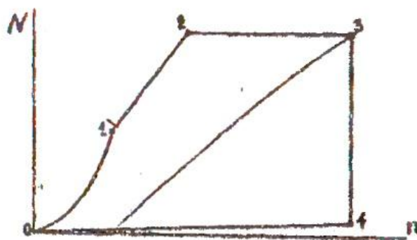
Рис. 6. Внешняя характеристика гидравлического тормоза
