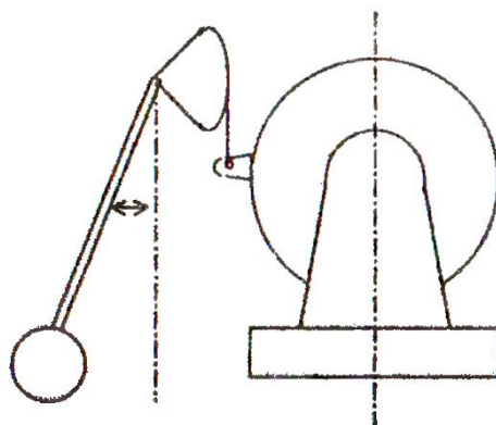
Рис. 7. Схема маятниковых весов
