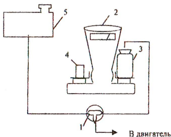
Рис. 8. Схема устройства для намерения расхода топлива
