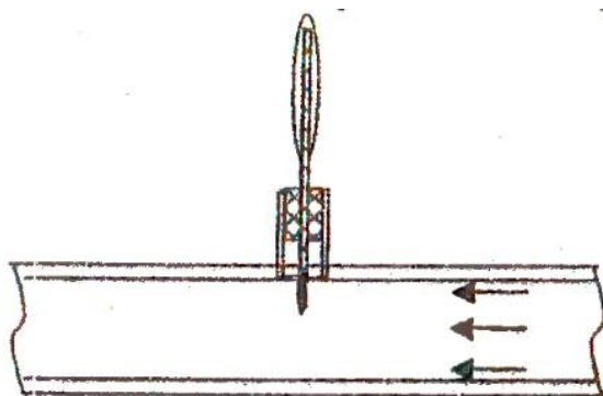
Рис. 11. Схема измерения температуры охлаждающей жидкости
