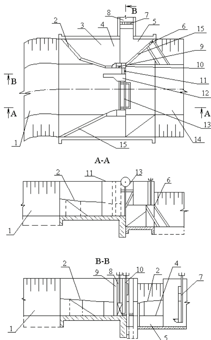
Рисунок 1 – Компонентная схема автоматизированного водозаборного гидроузла с щитовым отверстием для зимнего водоотбора с постоянным промывом наносов и отводом ледовошуговых образований:
