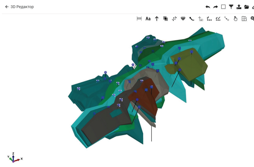
Рисунок 4 – Рудное тело, скважины
