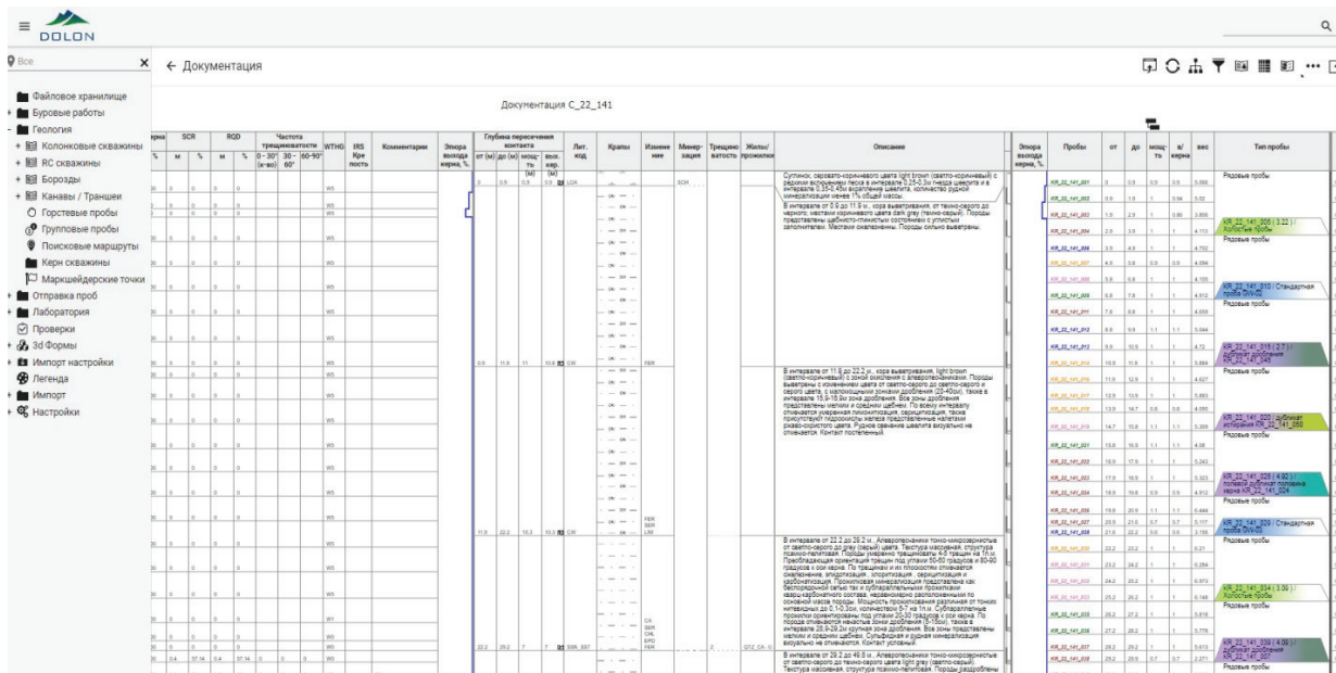
Рисунок 1 – Геологическая колонка
