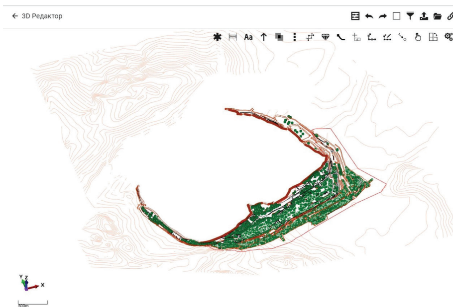
Рисунок 2 – Визуализация топоосновы с помощью изолиний и облако точек
