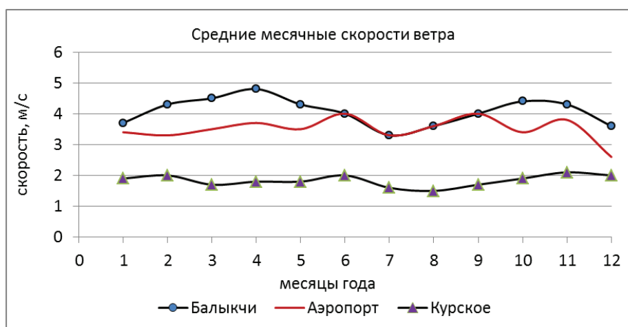
Рисунок 3 – Графики годового хода средних месячных скоростей ветра в АП Иссык-Куль за 2017 г. и на станциях Балыкчи и Курское [3]
