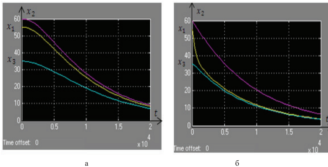
Рисунок 6 – Графическое представление зависимостей, полученных в компьютерной модели (а) и аналитическим методом (б); X1 – обмотка (желтый); X2 – магнитный проводник (фиолетовый); X3 – трансформаторное масло
