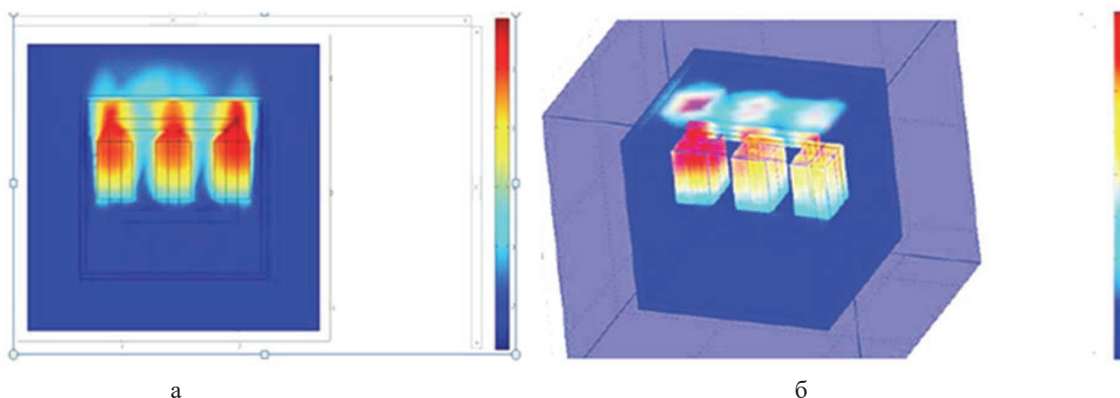
Рисунок 3 – Повышение температуры масла в верхнем слое обмотки: а – распределение теплового поля в КМТ без трехфазного дефекта; б – распределение теплового поля в КМТ с каким-либо дефектом в трехфазной фазе А (первая левая обмотка) [2, 3]
