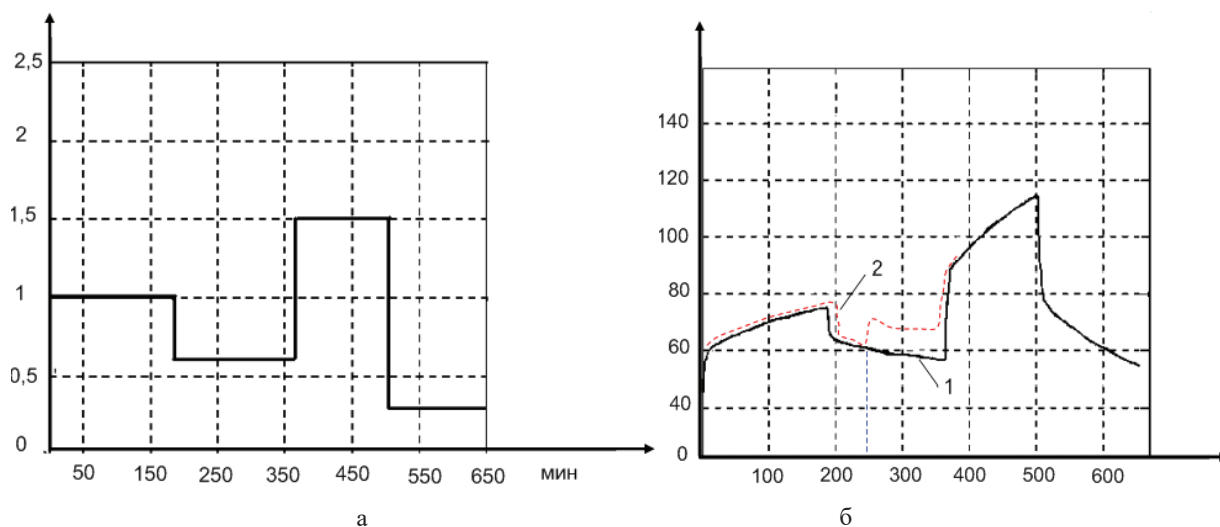
Рисунок 5 – Результат сравнения динамики изменения температуры: а – график нагрузки; б – график температуры в верхних слоях масла над обмоткой. 1 – нагрузка замены масла в верхних слоях масла над обмоткой, соответствующая графику; 2 – несоответствующая смена
