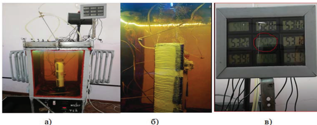
Рисунок 2 – Экспериментальный стенд силового масляного трансформатора [1]
