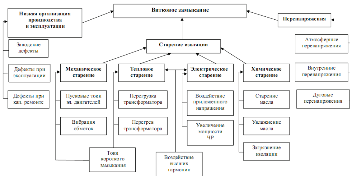
Рисунок 1 – Классификация факторов, влияющих на возникновение межконтурного скачка напряжения в обмотках трансформаторов 6–10/04 кВт
