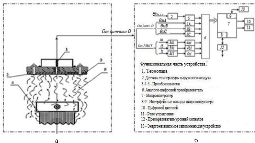
Рисунок 4 – Температура масла в верхних слоях обмоток датчика: а – установка и схематическое описание датчика измерения температуры: 1 – термопара; 2 – стеклотекстолит; 3 – фольга из меди; 4 – восходящий поток нагретого масла; 5 – обмотка трансформатора; б – функциональная схема термоматчика
