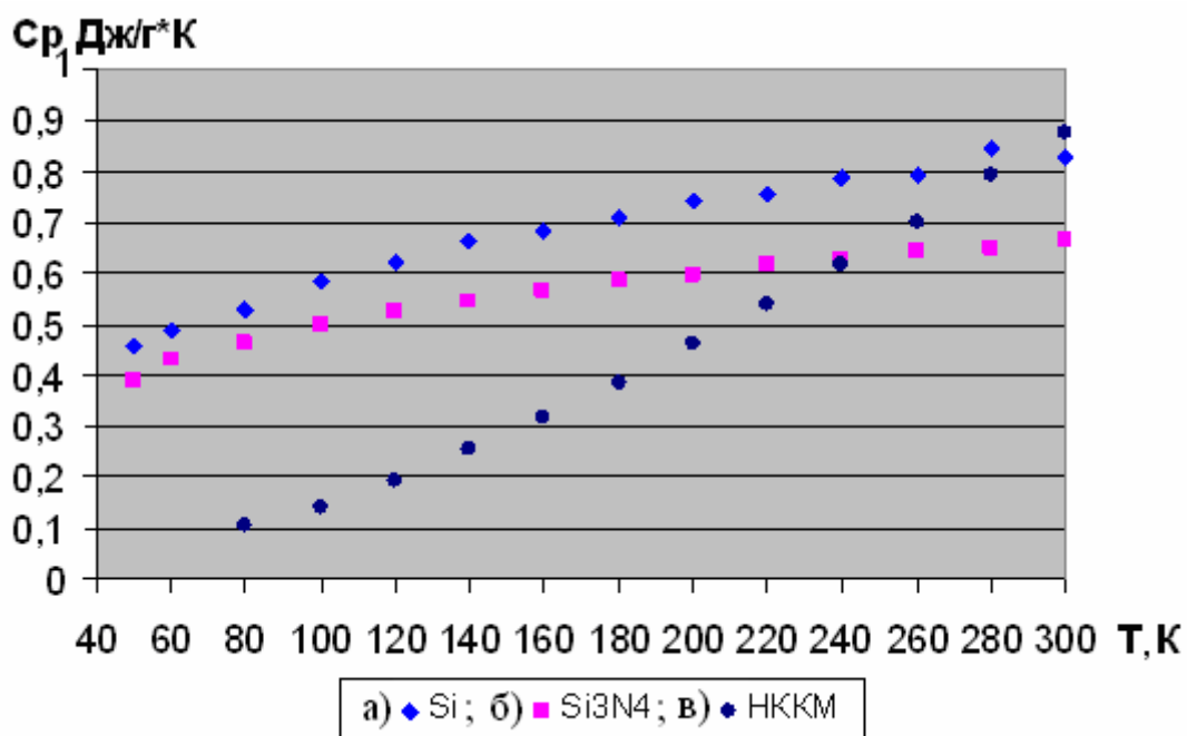
Рис. 1. Кривые зависимости теплоемкости от температуры: а- кремний Si (99,9999 %) [1,3], б- чистый нитрид кремния \text{Si}_3\text{N}_4 [1,3], в- ККМ из шламовых отходов КХМЗ “Астра”.
