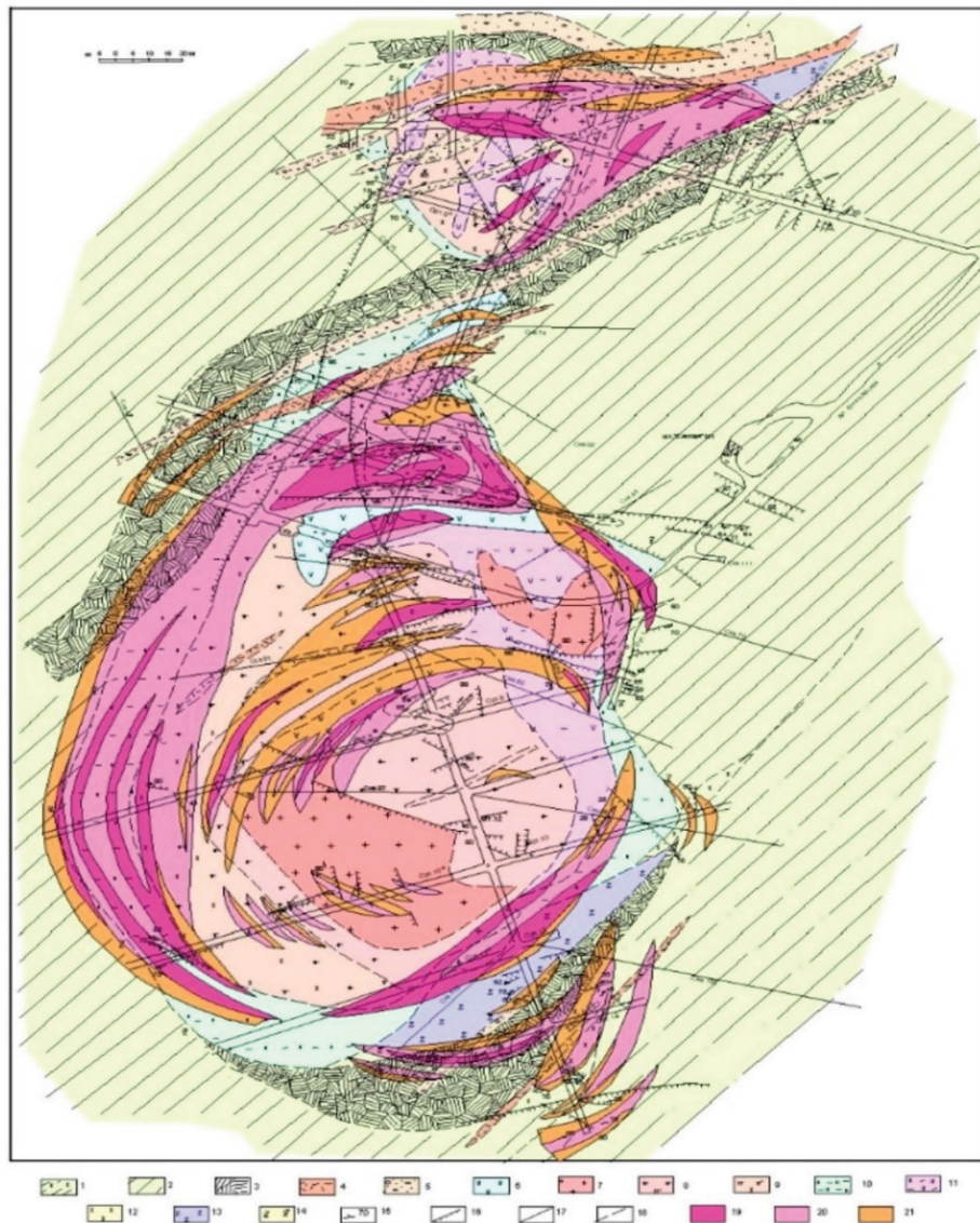
Рисунок 6 – Схема расположения редкоземельной минерализации на горизонте 2353 м месторождения Кутессай II. (Составители: Н.Н. Малокова, В.Ф. Ким, 2004 г.): 1 – гнейсы; 2 – зеленые амфиболовые сланцы; 3 – брекчированные амфиболовые сланцы; 4 – диабазовые порфириты; 5 – андезитовые порфириты; 6 – догранофировый кварц; 7 – гранофиры; 8 – кварц-серцитовый метасоматит; 9 – кварц-хлорит-серцитовый метасоматит; 10 – кварц-хлоритовый метасоматит; 11 – вторичный кварц; 12 – кварц-полевошпатовый метасоматит по гнейсу; 13 – биотит-хлоритовые и биотитовые роговики; 14 – контактовые роговики; 15 – элементы залегания; 16 – тектонические нарушения; 17 – прослеженные контакты пород; 18 – интерполированные контакты пород; 19 – участки с содержанием карбонатов и фтор-карбонатов редких земель более 1%; 20 – участки с содержанием карбонатов и фтор-карбонатов редких земель более 0,01 до 0,1%; 21 – участки с содержанием карбонатов и фтор-карбонатов редких земель более 0,01 до 0,01 %
