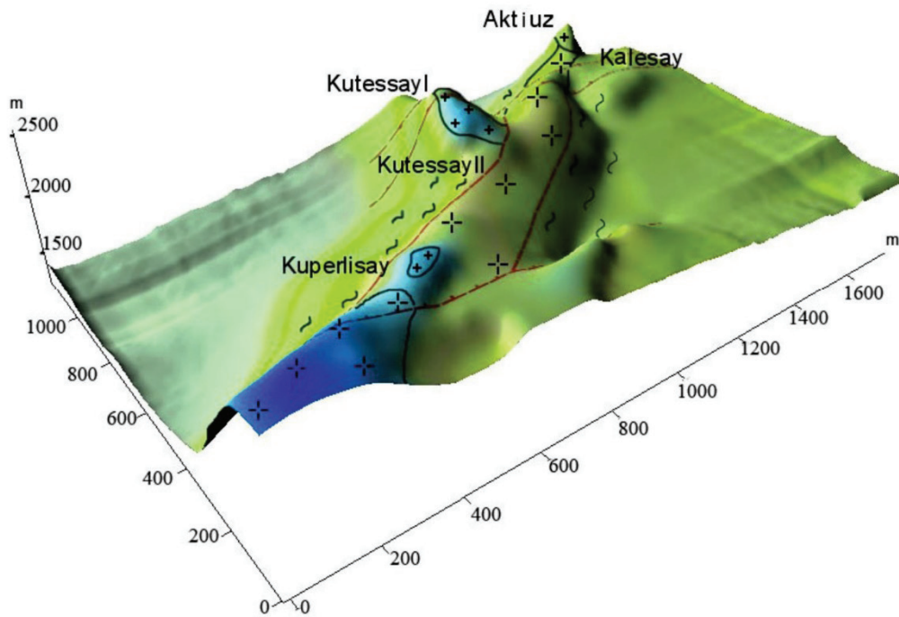
Рисунок 2 – Структура размещения месторождений в Актюзском рудном поле и рудоносных гранофиров, секущих Куперлисайскую трещинную интрузию
