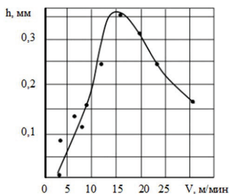
Рисунок 5 – Зависимость высоты нароста на уголках сверла от скорости резания
