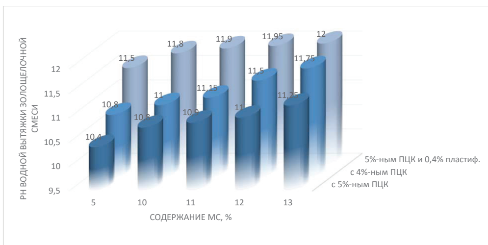
Рисунок 2 – Изменение pH водной вытяжки золощелочной смеси в зависимости от МС
