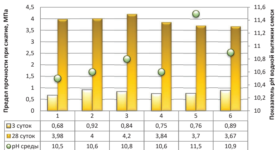
Рисунок 1 – Зависимости прочности на сжатие от составов смесей и pH водной вытяжки
