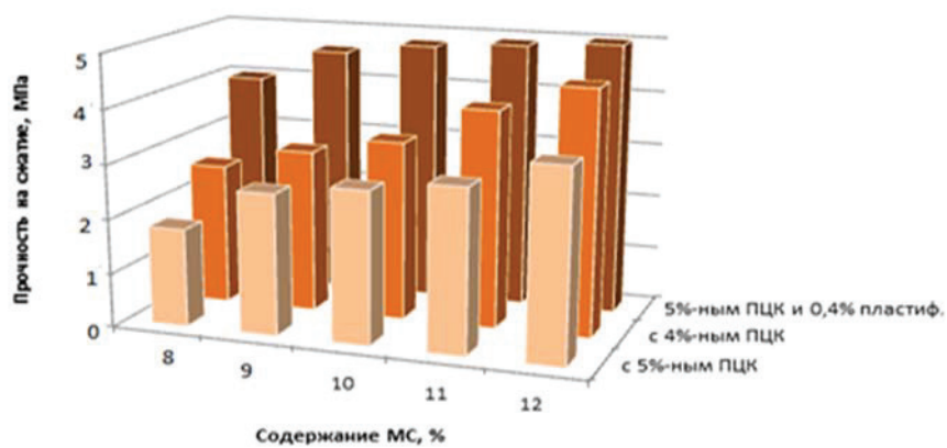
Рисунок 3 – Изменение прочности золосодержащего вяжущего в зависимости от добавки МС
