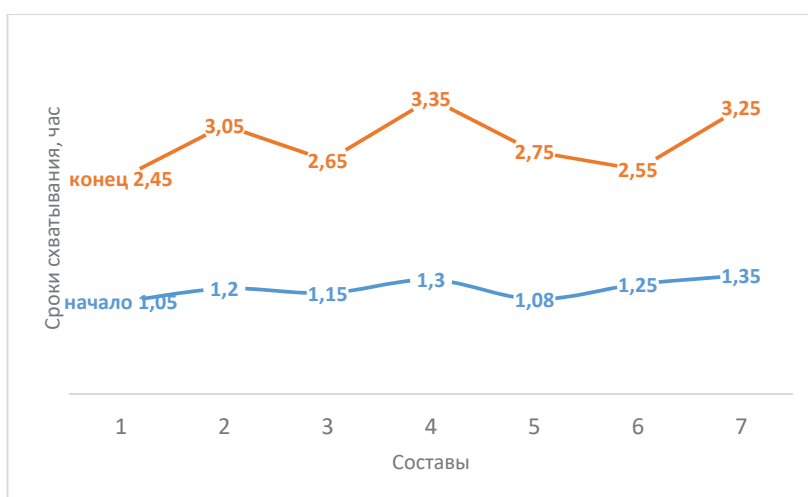
Рисунок 4 – Сроки схватывания гипсозолощелочных вяжущих композиций (среднестатистические данные)
