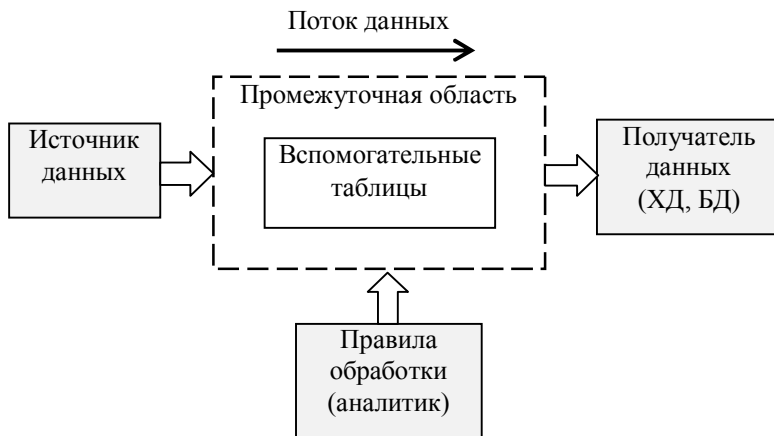
Рис. 1. Поток данных в ETL
