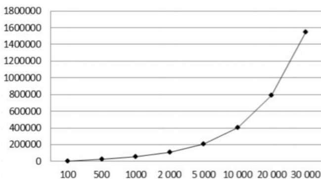
Рис.4. Зависимость времени последовательной обработки от количества записей
