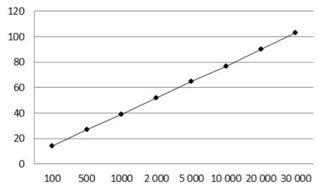
Рис.5. Зависимость времени параллельной обработки от количества записей
