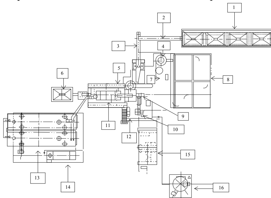
Рис. 7. Технологическая схема завода для приготовления асфальтобетона с применением золы-уноса: 1-предварительные дозаторы минеральных материалов; 2-ленточный конвейер; 3-конвейер для агрегатов; 4-пылесборник; 5-сортировочно-смесительный агрегат; 6 - бункер для минерального порошка; 7-вытяжной вентилятор; 8-бассейн для выбросов; 9-горячий элеватор; 10-сушильный барабан; 11-миксер; 12-воздушный компрессор; 13 – цистерна для битума; 14-масляная грелка для битума; 15-кабина управления установкой; 16-дизельный генератор.
