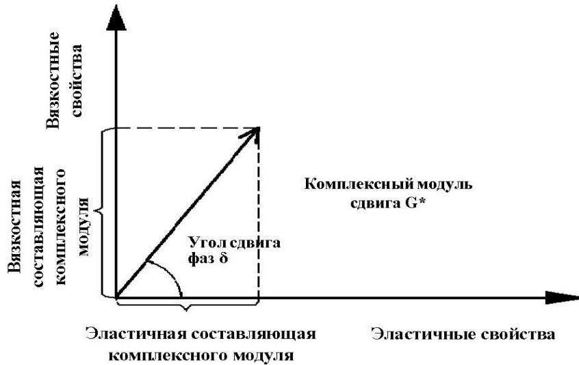
Рис.2. Схема-интерпретация комплексного модуля сдвига
