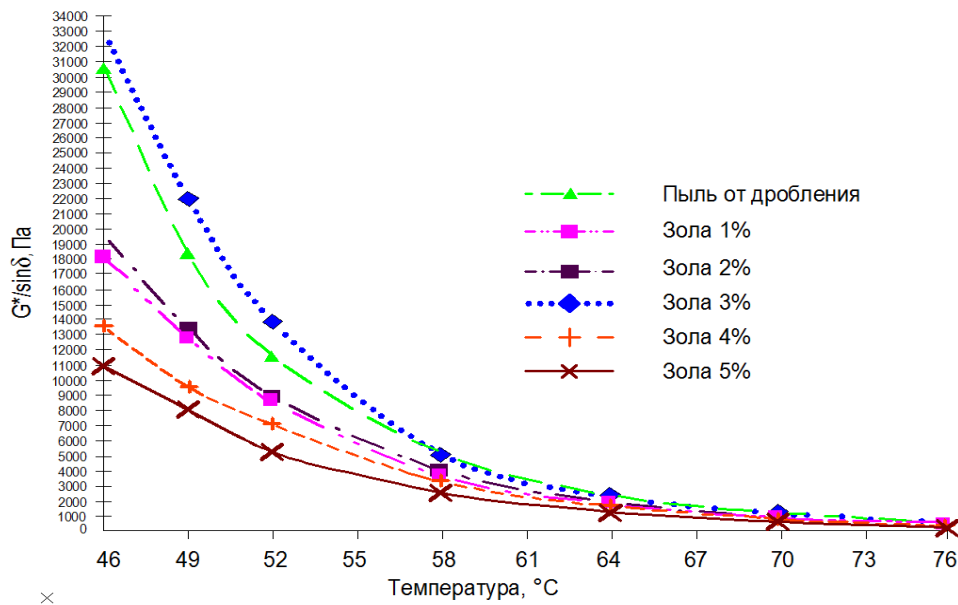
Рис. 4. Диаграмма показателей устойчивости асфальтобетона к колееобразованию с применением минерального порошка из золы-уноса
