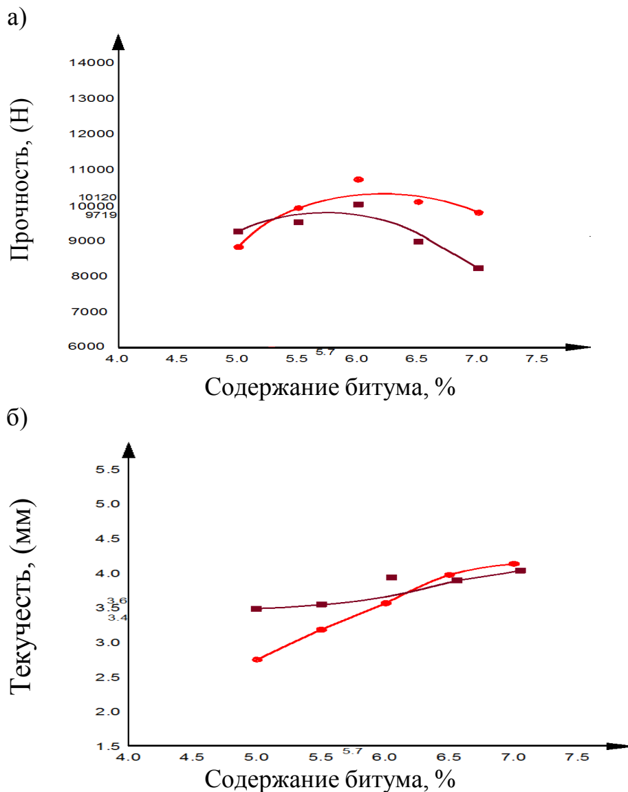
Рис.6. Кривые результатов испытаний образцов уплотненных горячих асфальтобетонных смесей по методу Маршалла:
