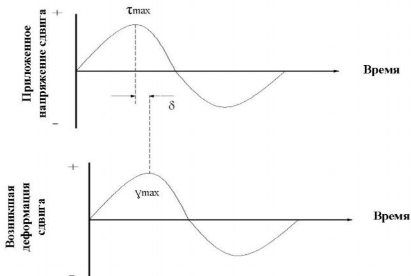
Рис.1. Кривые приложенных напряжений сдвига и возникающих деформаций
