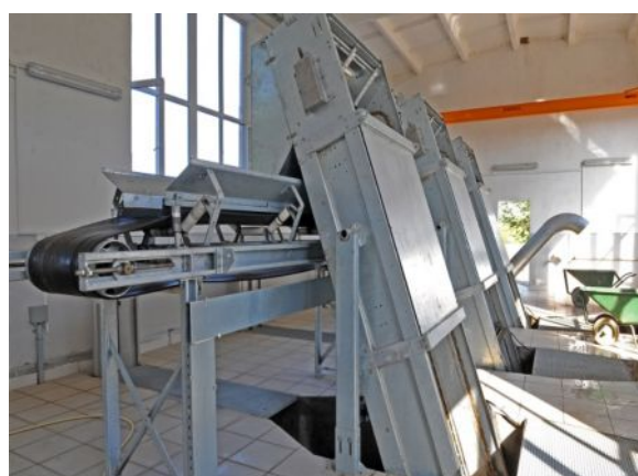
Рис.2. Решетки очистного сооружения г.Ош после реконструкции
