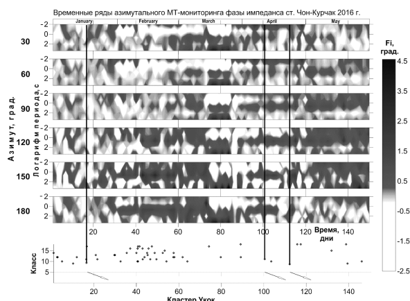
Рисунок 7 – Результаты МТ-мониторинга (ЧВР вариаций фазы импеданса) по данным станции Чон-Курчак в сопоставлении с сейсмичностью Укокского кластера за январь–май 2016 г. (ромбики – сейсмические события)
