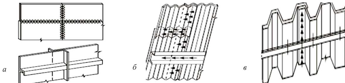
Рисунок 1 – Металлические панели: а – из гладких листов; б – из волнистых листов; в – из гофрированных листов
