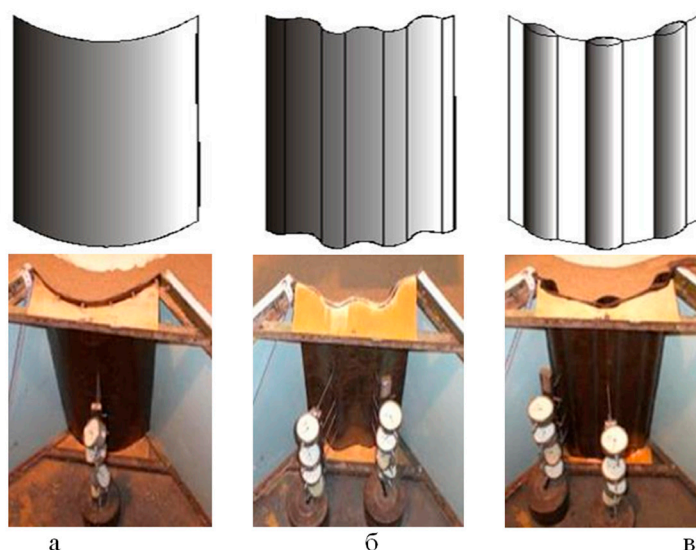
Рисунок 2 – Металлические панели: а – гладкая; б – волнистая; в – ребристая
