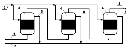
Рисунок 2 – Технологическая схема локальной очистки сточных вод: 1 – подача сточной воды; 2 – подача сорбента; 3 – отвод очищенной воды; 4 – фильтры адсорбционные; 5 – отвод отработанного сорбента
