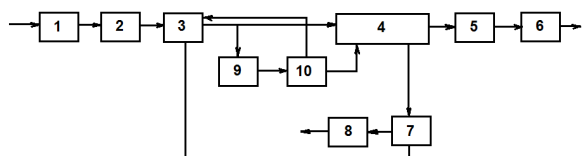
Рисунок 1 – Технологическая схема системы доочистки сточных вод: 1 – приемная емкость; 2 – насосная установка 3 – решетка; 4 – сорбционные фильтры; 5 – хлоратор (при необходимости); 6 – быстроток-аэратор; 7 – емкость для промывки вод; 8 – насос; 9 – резервуар для промывки решеток и фильтров; 10 – насос для подачи воды на промывку
