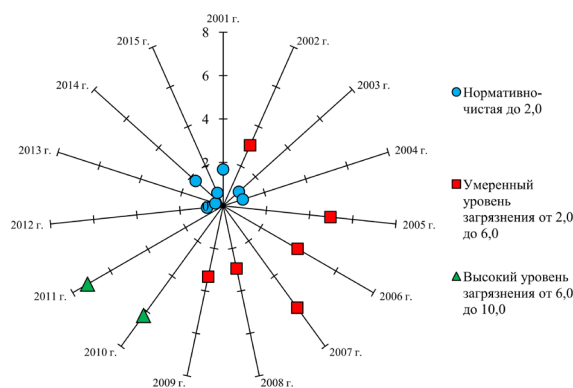
Рисунок 1 – Оценочные показатели загрязнения Капшагайского водохранилища по результатам КИЗВ с учетом класса опасности
