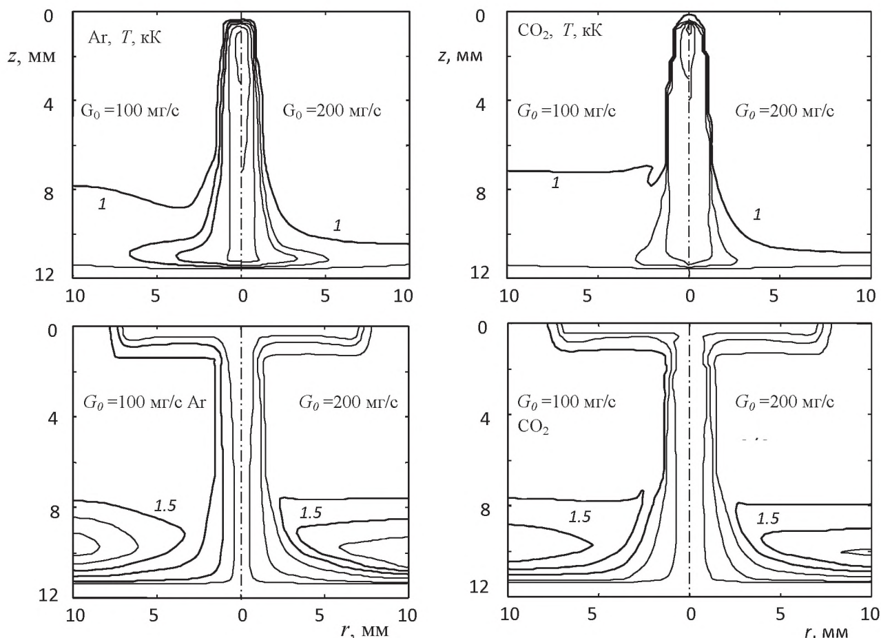
Рис. 1. Линии тока газа ( G/G_0=0.05, 0.3, 0.9, 1.5, 2, 2.5 ) и изотермы дуги ( T=1, 5, 10, 15, 20 кК) в аргоне и в углекислом газе; I=70 А.
