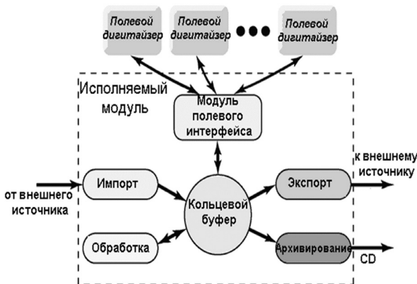
Рисунок 7 – Система Antelope передачи потока данных в режиме реального времени
