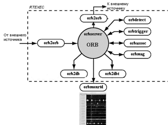
Рисунок 8 – Структура процесса RTEXC на Научной станции РАН
