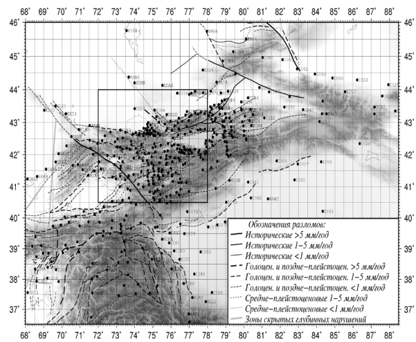
Рисунок 2 – Расположение пунктов наблюдений ЦА GPS-сети, для которых получена оценка вектора скорости современного движения. Прямоугольником выделена зона, рассматриваемая в данной работе
