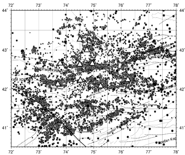
Рисунок 1 – Эпицентральное расположение сейсмических событий (круги, размер – магнитуда) и станций сети KNET (треугольники). Линиями на этом и последующих рисунках показаны разломы по [11]
