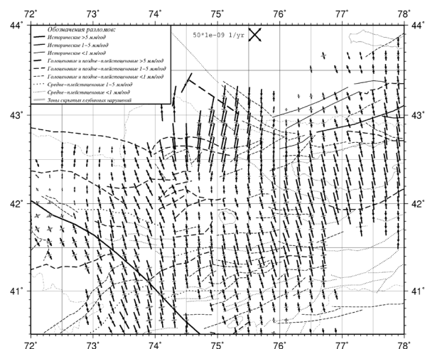
Рисунок 4 – Поле значений тензора скорости деформации земной коры, рассчитанное по данным GPS-наблюдений. Черный цвет показывает сжатие, серый – растяжение
