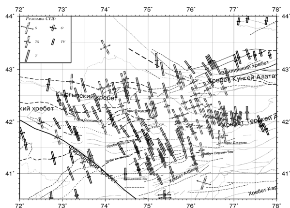
Рисунок 3 – Карта сейсотектонических деформаций. Прямоугольником обозначено направление оси сжатия, стрелочками – направление оси растяжения. Длина прямоугольника и стрелочек определяется проекцией оси сжатия и растяжения на горизонтальную плоскость
