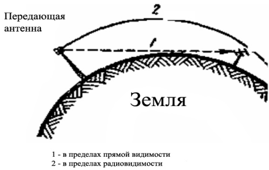
Рисунок 1 – Распространение ультракоротких волн
