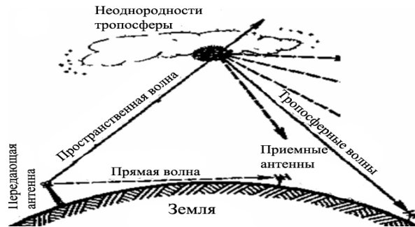
Рисунок 2 – Распространение ультракоротких волн за счет рассеяния в тропосфере
