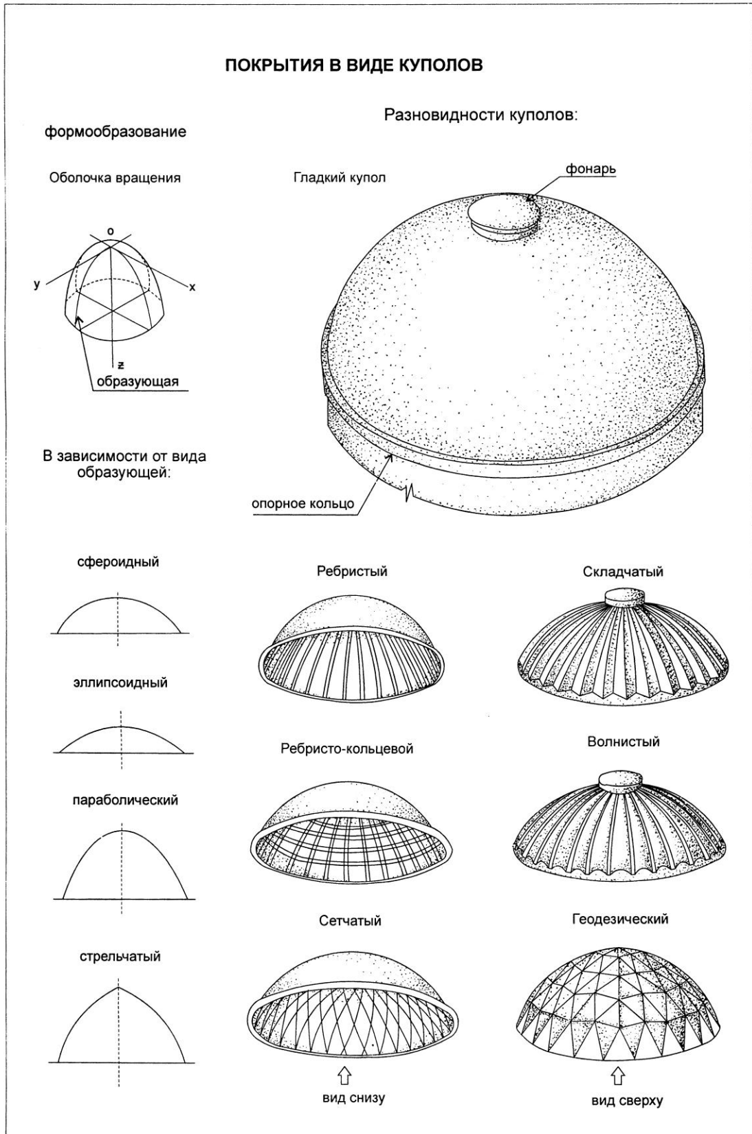
Рис. 2. Типы купольных покрытий зальных помещений [4]
