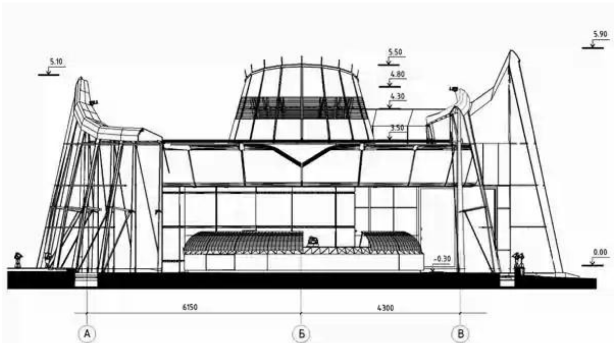
Рис.8. РАЗРЕЗ 1-1
