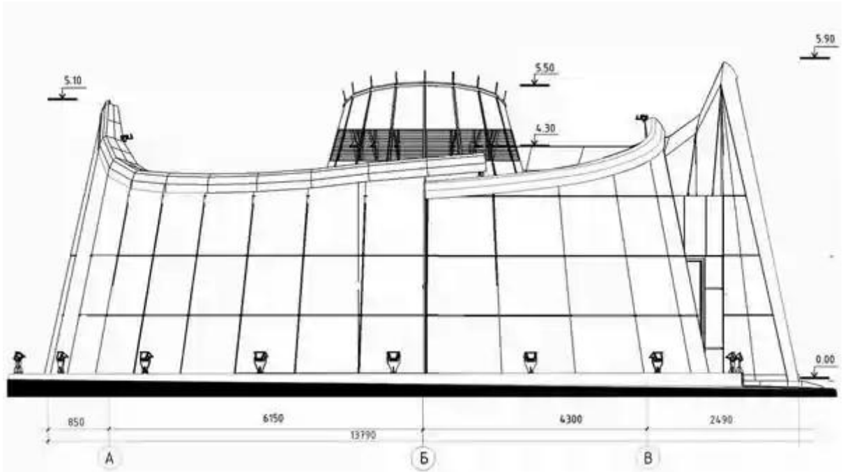
Рис.7. ФАСАД В ОСЯХ А-В
