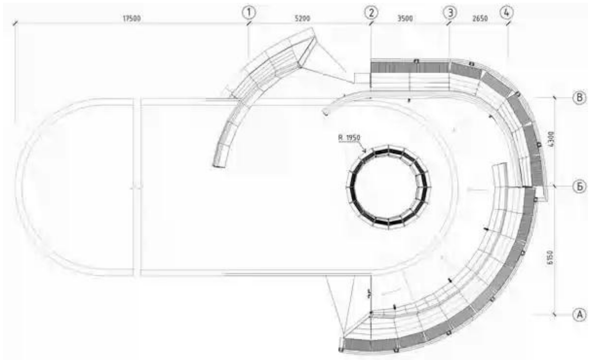
Рис.9. ПЛАН КРОВЛИ
