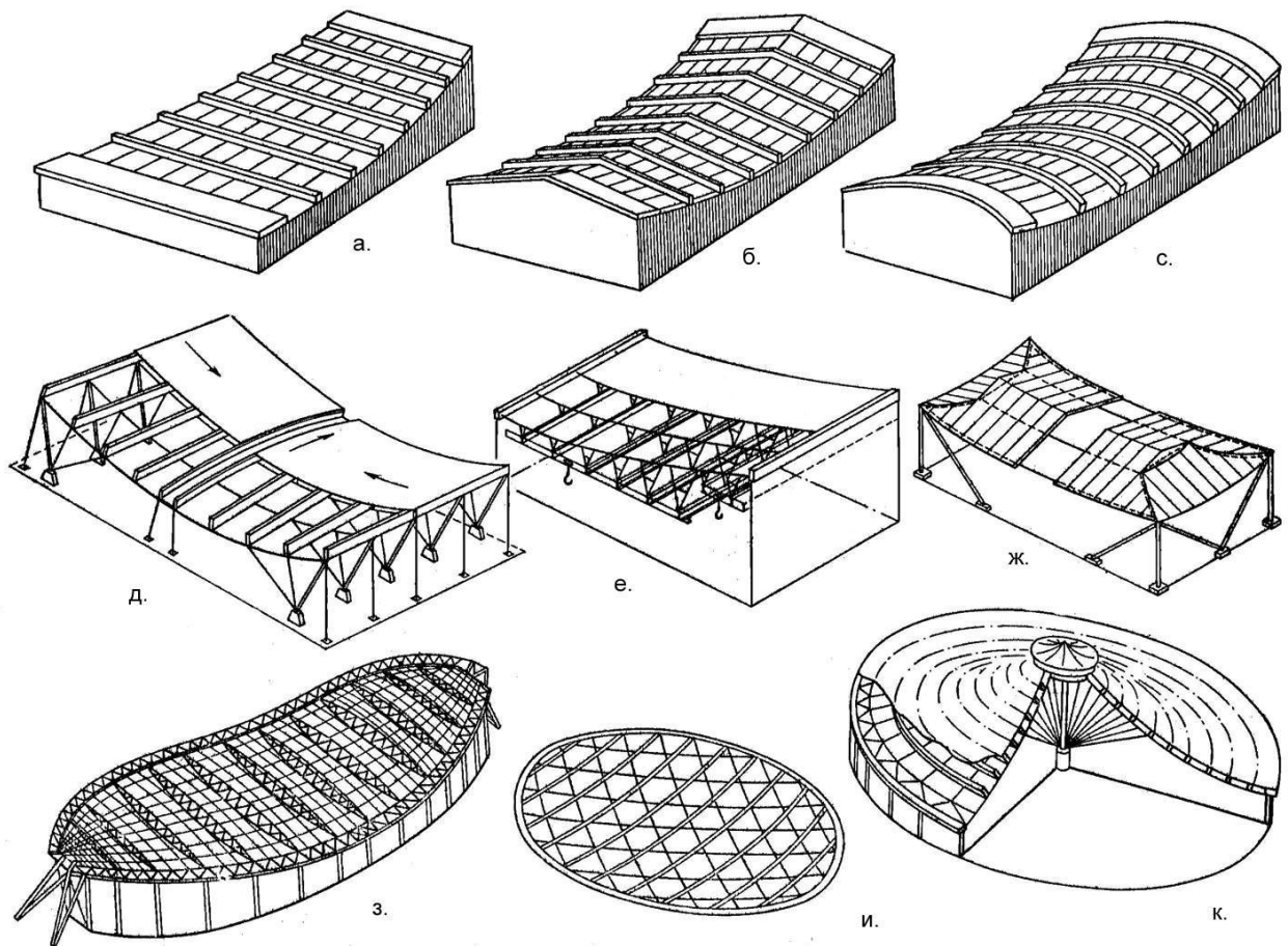
Рис. 5. Конструктивные формы комбинированных висячих покрытий [4]:
