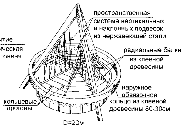
С опорами в виде трех наклонных пилонов
