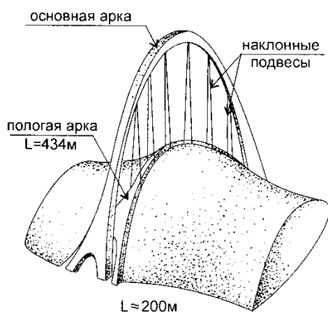
Рис. 4. Принципиальные схемы подвесных покрытий зальных помещений [4]
