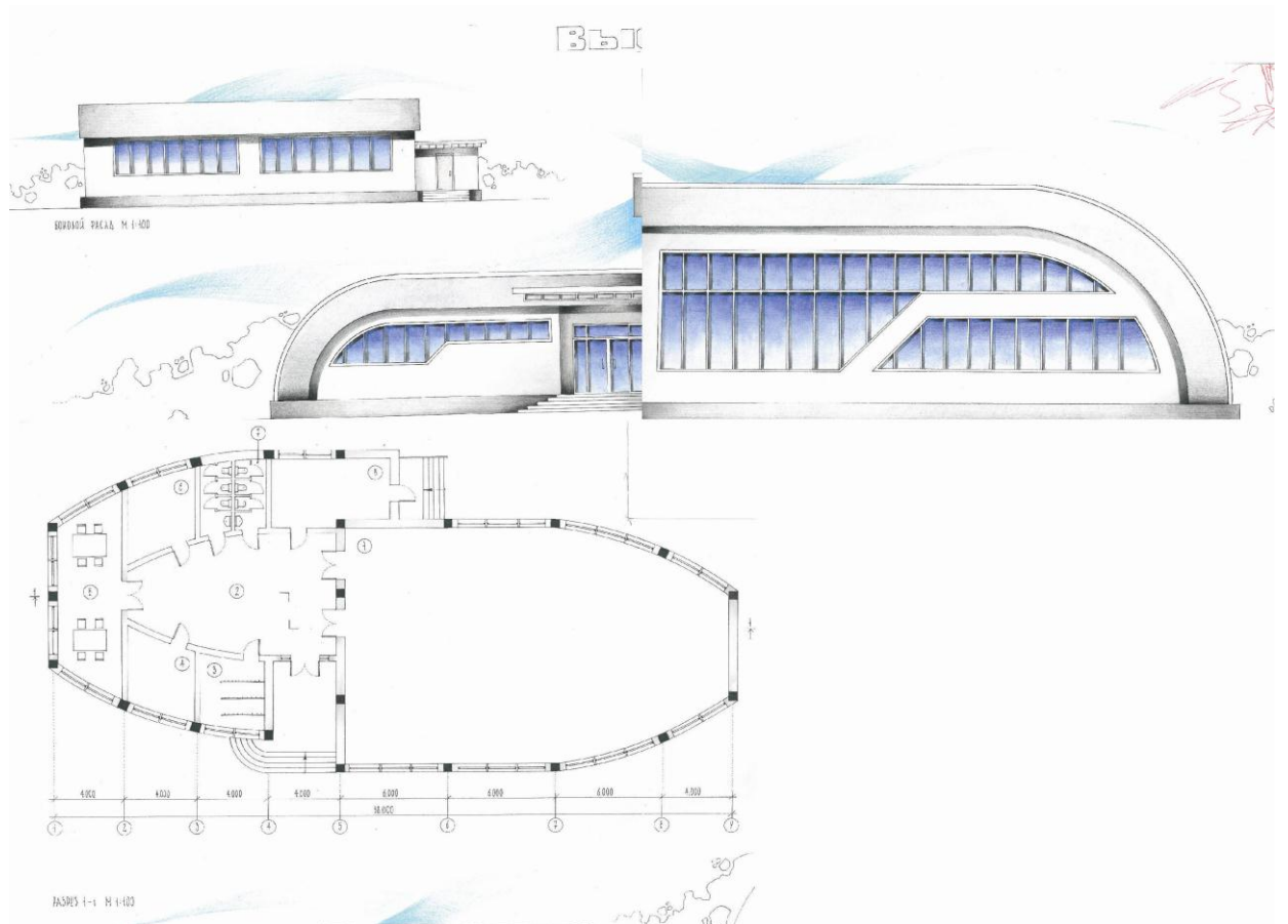
Рис.13. Пример курсового проекта выставочного павильона. Авт.ст. гр. Арх-1-10 М. Будунова. Фасады и план
