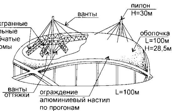
Рис. 4. Принципиальные схемы подвесных покрытий зальных помещений [4]
