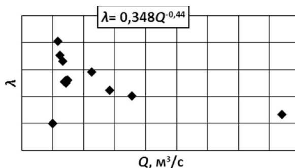
Рисунок 7 – График зависимости коэффициентов гидравлического сопротивления \lambda от расходов Q
