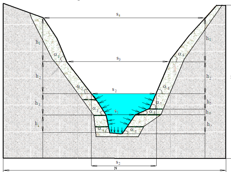
Рис.3. Геометрические параметры склонов неоднородного сложения
