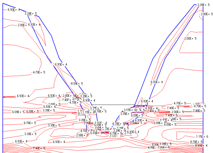
Рис.6. Распределение горизонтальных напряжений в массиве склонах неоднородного сложения при уровне воды 130м.
