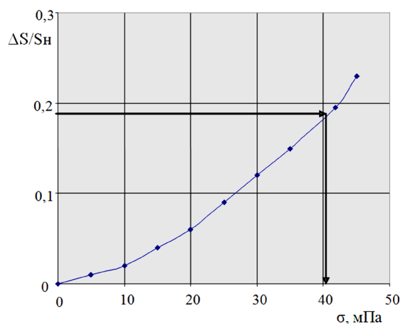
Рисунок 4 – Определения напряжений в элементах металлических конструкций по тарировочной кривой
