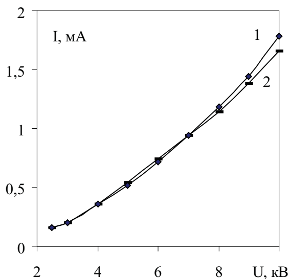
Рис. 2. Вольт-амперная характеристика разряда: 1 – разряд внутри ПНП, 2 – разряд снаружи ПНП.
