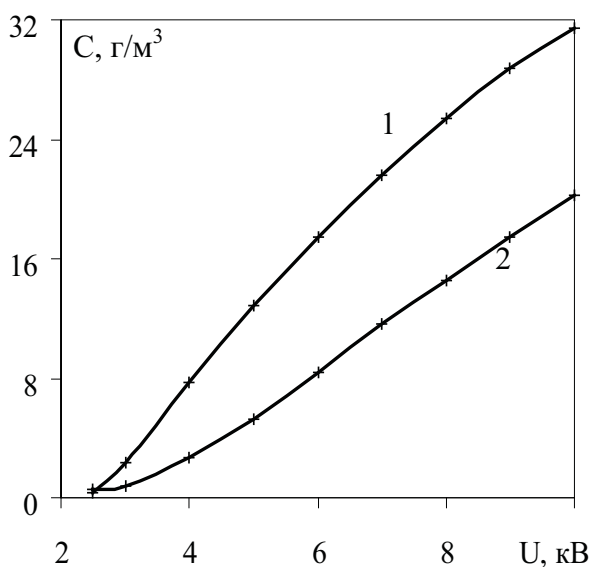
Рис. 3. Концентрация озона в разряде: 1 – снаружи ТУТ, 2 – внутри ТУТ.
